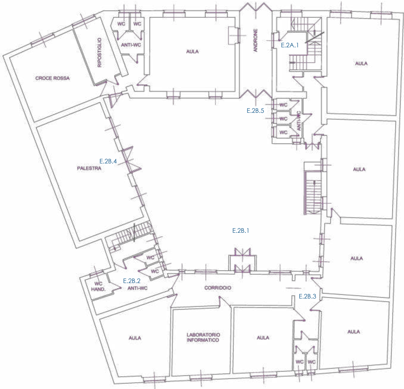
E.2A-2B Pianta Piano Terra
